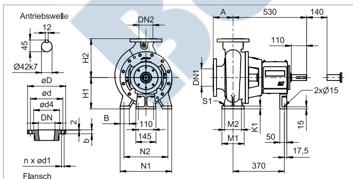
Type BPP 100-250 - BPP 125-400
