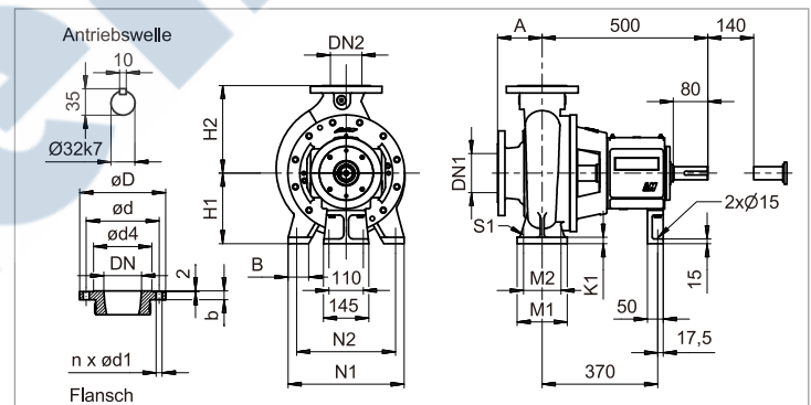
Type BPP 065-200 - BPP 50-315
