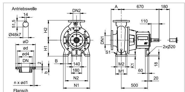
Type BPP 200-250 - BPP 200-400
