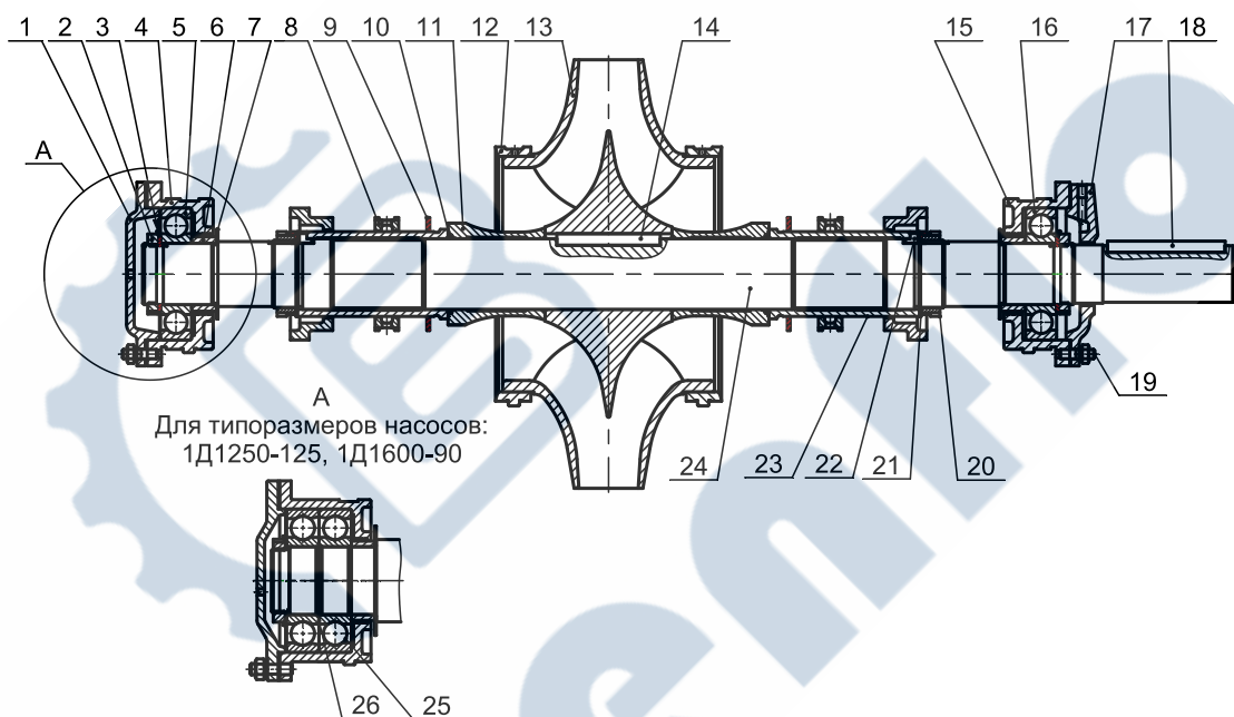
Рисунок 2 - Ротор насоса с сальниковым уплотнением
