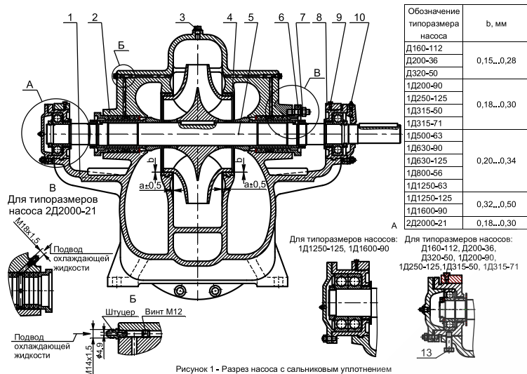
Рисунок 1 - Разрез насоса с сальниковым уплотнением
