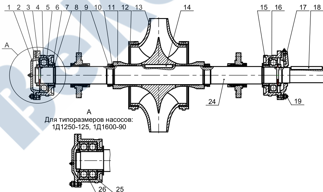
Рисунок 2.1 - Ротор насоса с торцовым уплотнением
