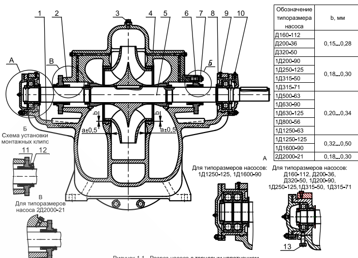
Рисунок 1,1 - Разрез насоса с торцовым уплотнением
